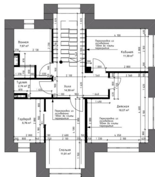
План возводимых конструкций 2 этажа
